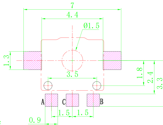
PCB焊板安装图示
